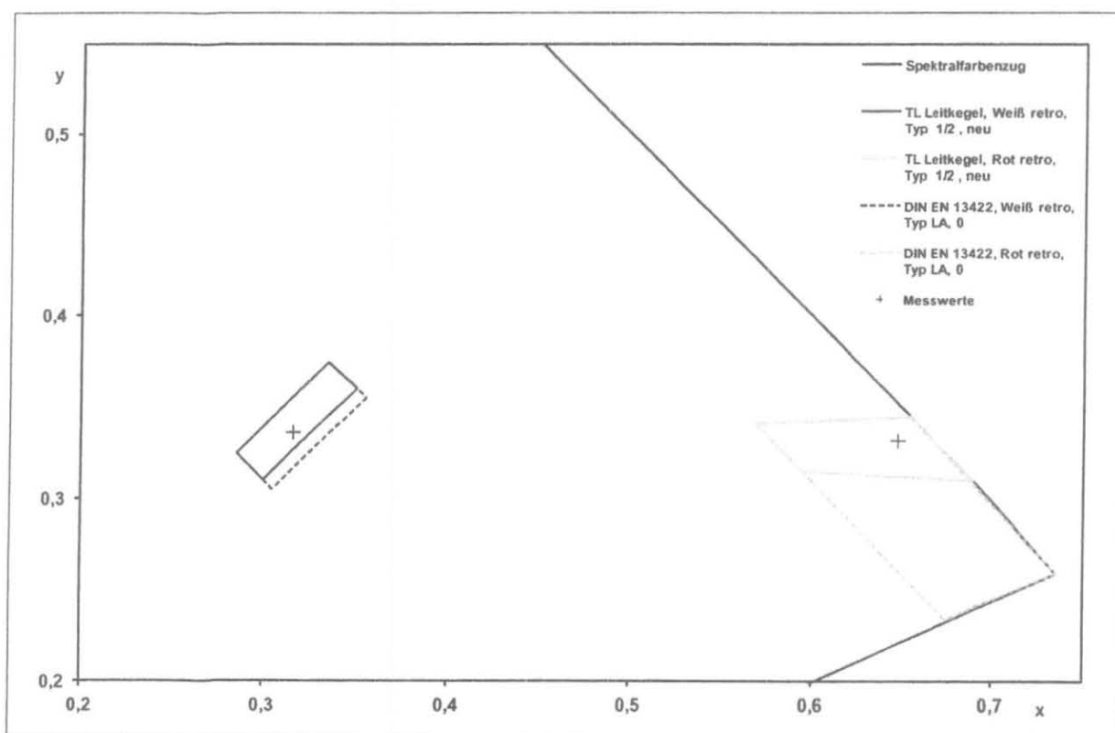
Bild 3: Farbort der retroreflektierenden Folie
