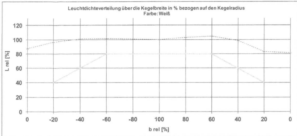
Bild 4: rel. Leuchtdichteverteilung über die Kegelbreite in % bezogen auf den Kegelradius (Weiß)
